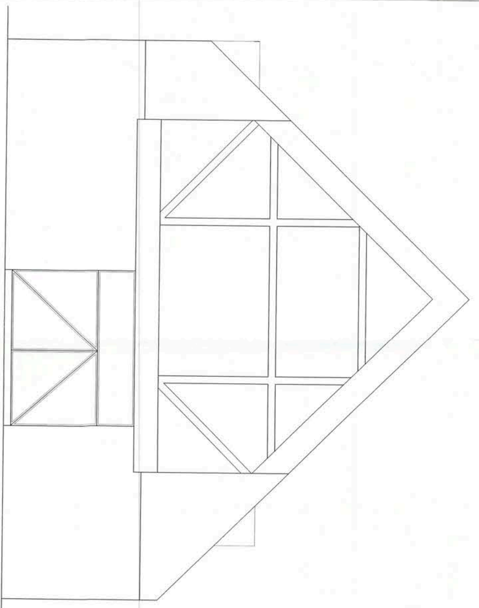
FACHADA FRONTAL ESC. 1:50
