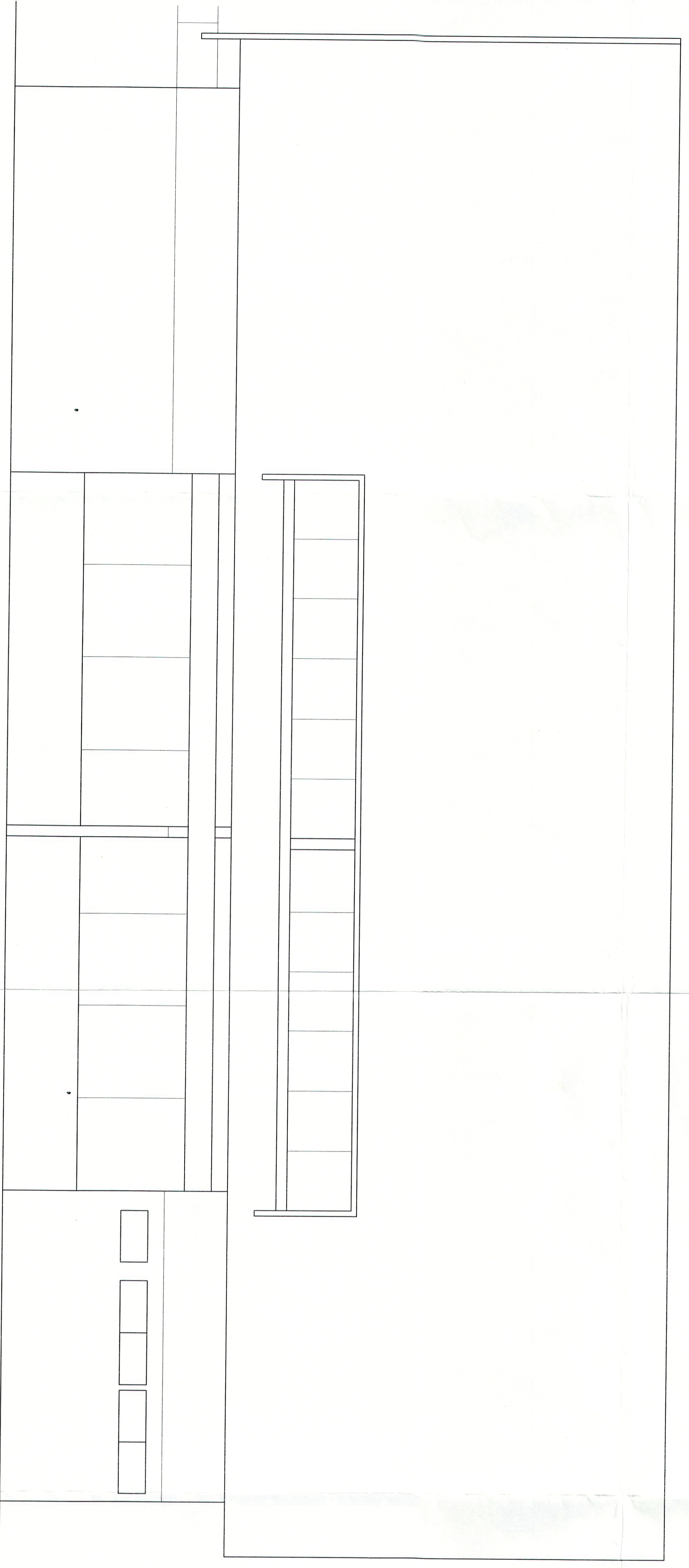
FACHADA LATERAL ESC. 1:50
